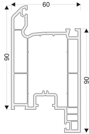
PRO04 Inward Door Profile
