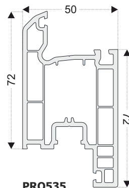
PRO535 Inward Door Profile
