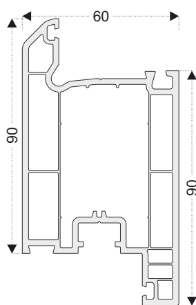
PRO004 Inward Door Profile
